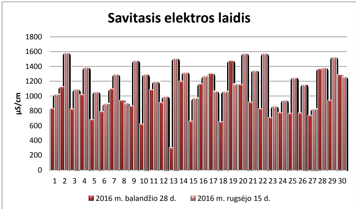
28 pav. Savitojo elektros laidžio koncentracija Joniškio rajono požeminiame vandenyje
