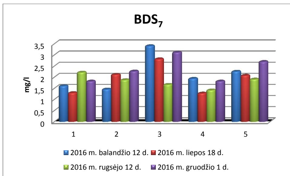
25 pav. BDS 7 koncentracija Jonišchio paviršiniuose vandens telkiniuose.
