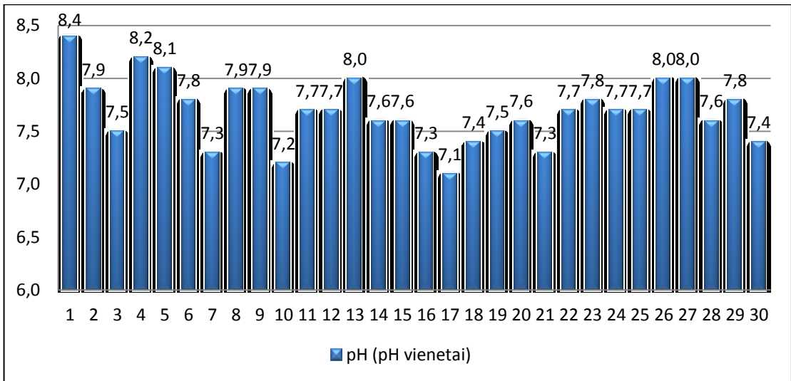
27 pav. pH koncentracija Joniškio rajono požeminiame vandenyje
