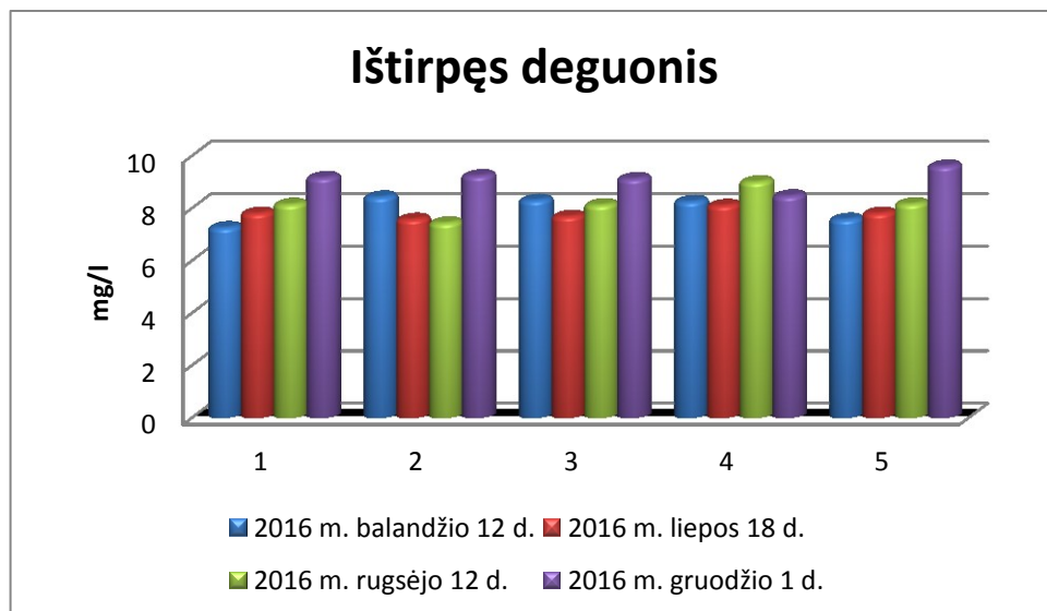
24 pav. Ištirpusio deguonies koncentracija Jonišchio rajono paviršiniuose vandens telkiniuose.
