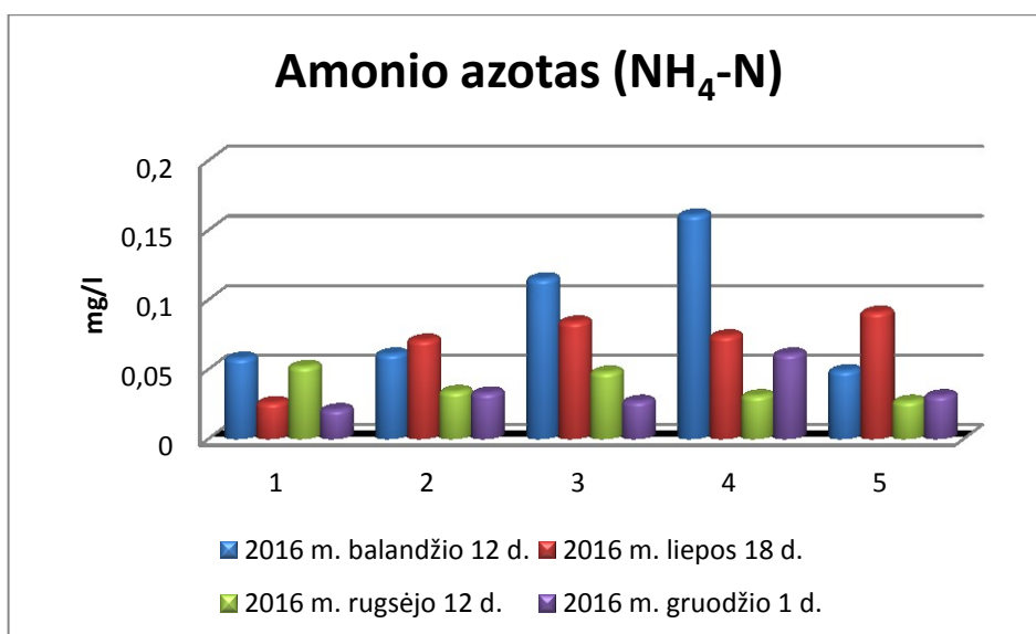
19 pav. Amonio azoto koncentracija Joniškio rajono paviršiniuose vandens telkiniuose.
