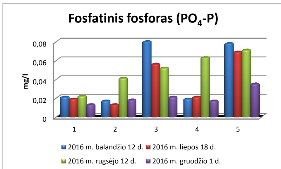
23 pav. Fosfatinio fosforo koncentracija Jonišchio rajono paviršiniuose vandens telkiniuose.
