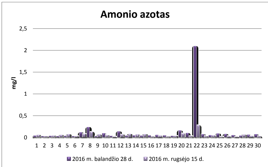
30 pav. Amonio azoto koncentracija Joniškio rajono požeminiame vandenyje
