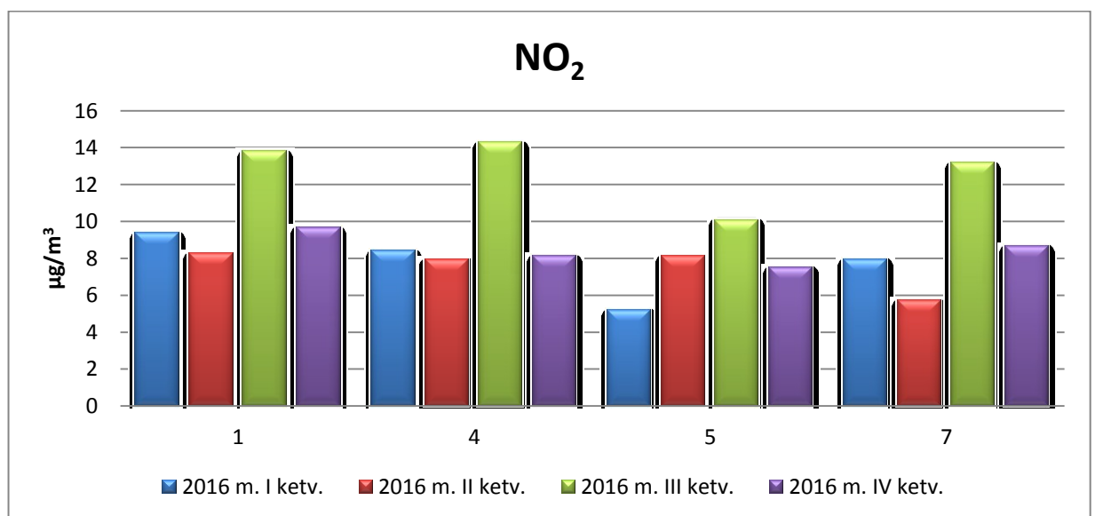
7 pav. NO 2 koncentracijų pasiskirstymai Joniškio rajone.
