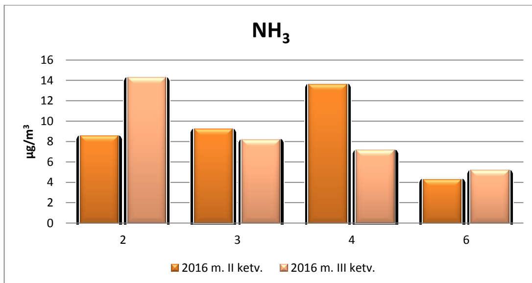
14 pav. NH 3 koncentracijų pasiskirstymas Joniškio rajone.
