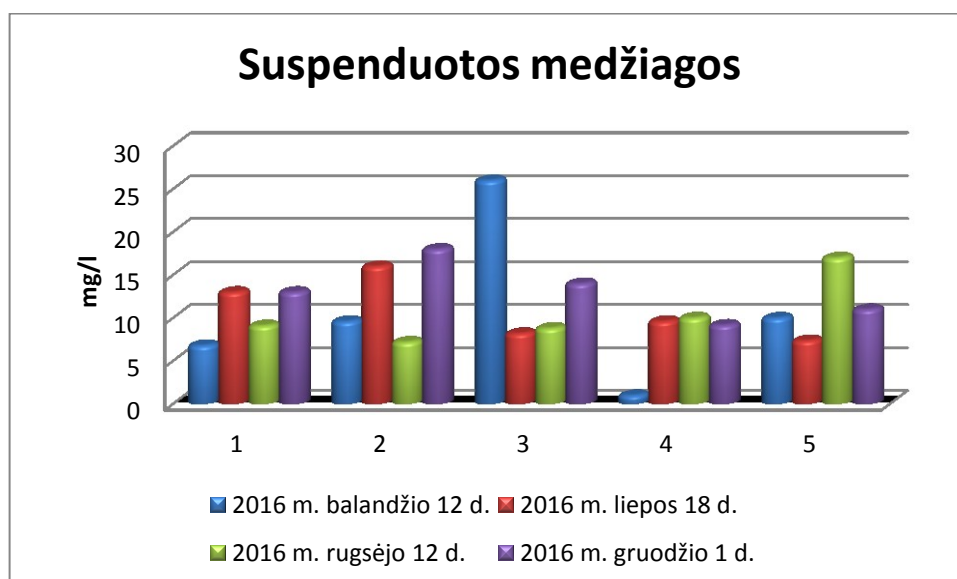
26 pav. Suspenduotų medžiagų koncentracija Jonišchio rajono paviršiniuose vandens telkiniuose.
