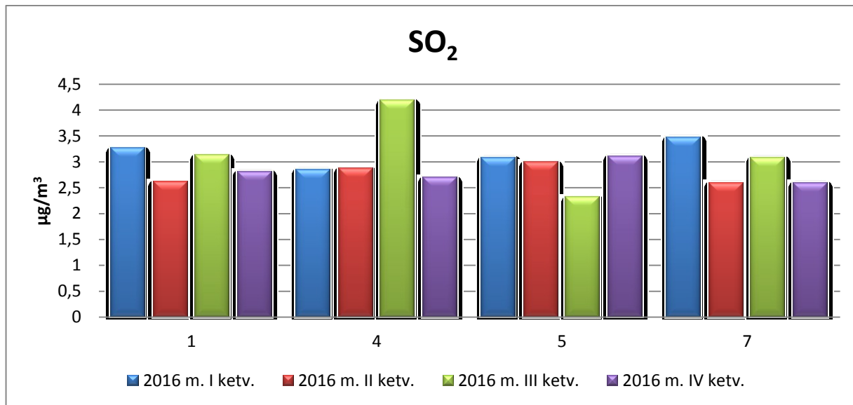
8 pav. SO 2 koncentracijų pasiskirstymai Joniškio rajone.
